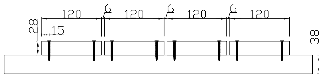
剖面圖 比例 1 : 4
